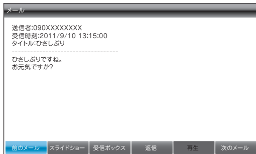
メール画面
