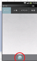
起動画面
